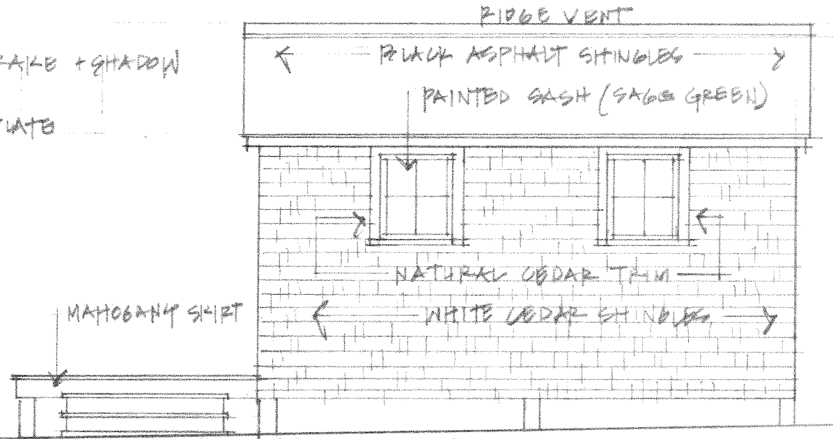
EAST ELEVATION (PATH)
