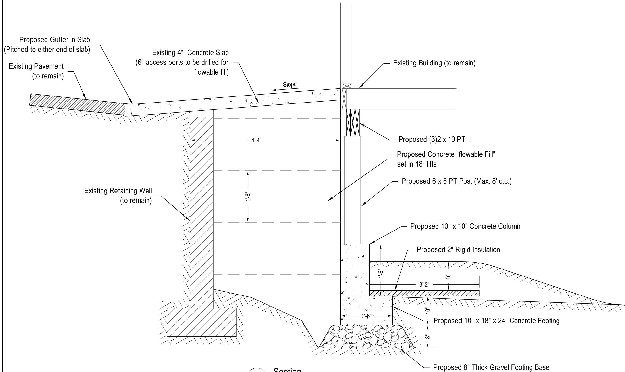
1 Section Scale: \frac{3}{4}'' = 1'-0''
